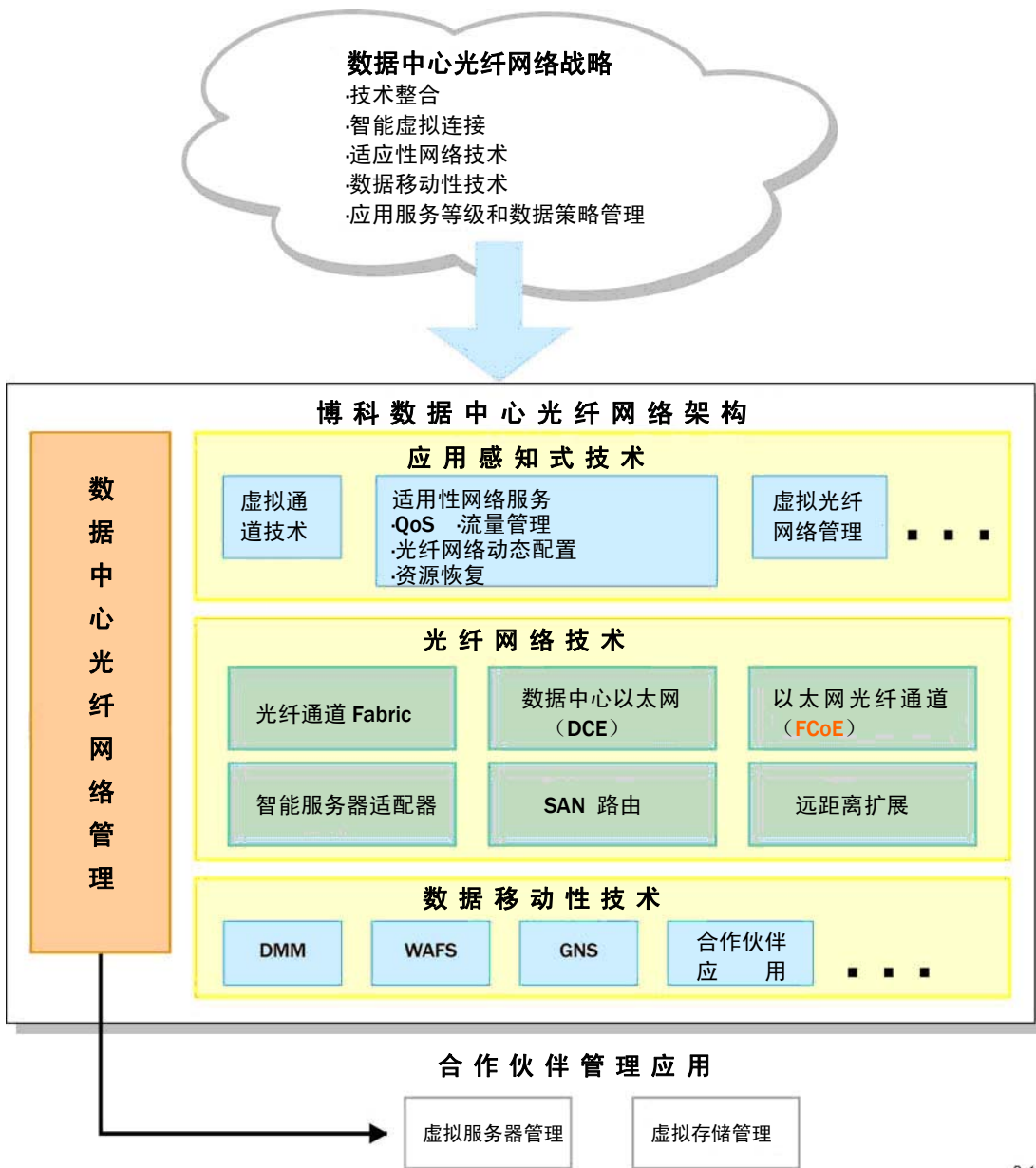
图 2. 博科数据中心光纤网络(DCF)架构
