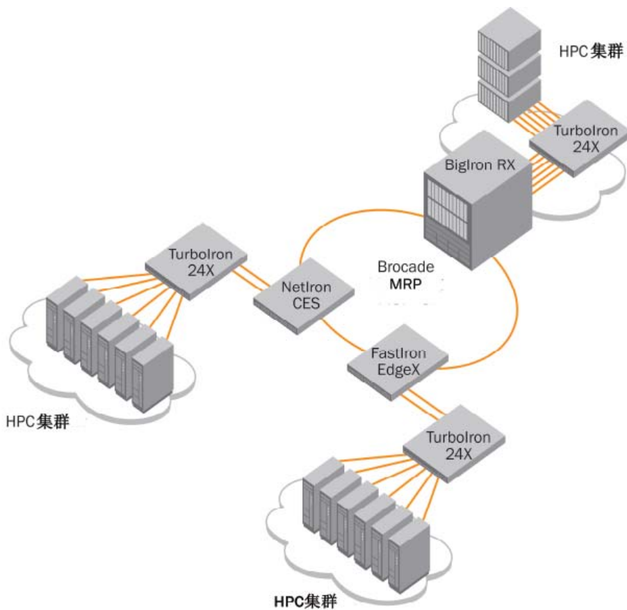
图4. Turbolron 24X提供HPC集群互联，而Brocade FastIron、NetIron和BigIron提供MRP连接。
