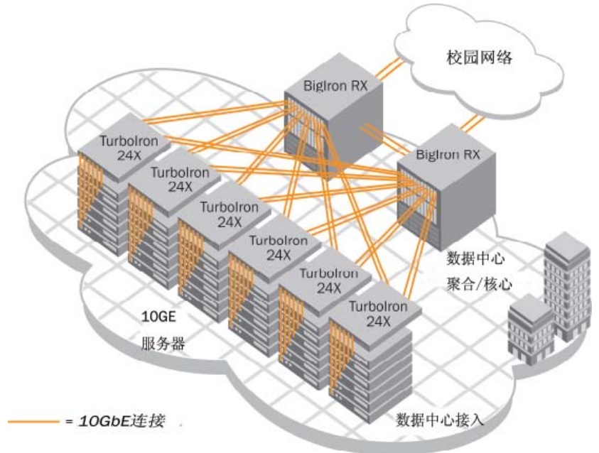
图2. Turbolron 24X用于提供数据中心架顶式交换机接入，而Brocade BigIron RX则提供聚合解决方案。
